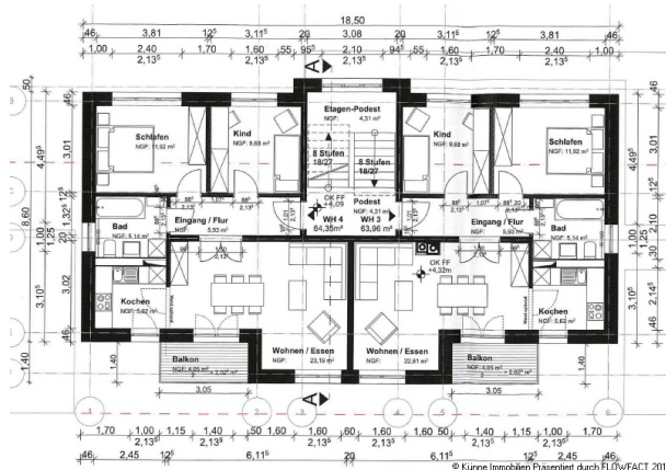
Grundriss Obergeschoss
