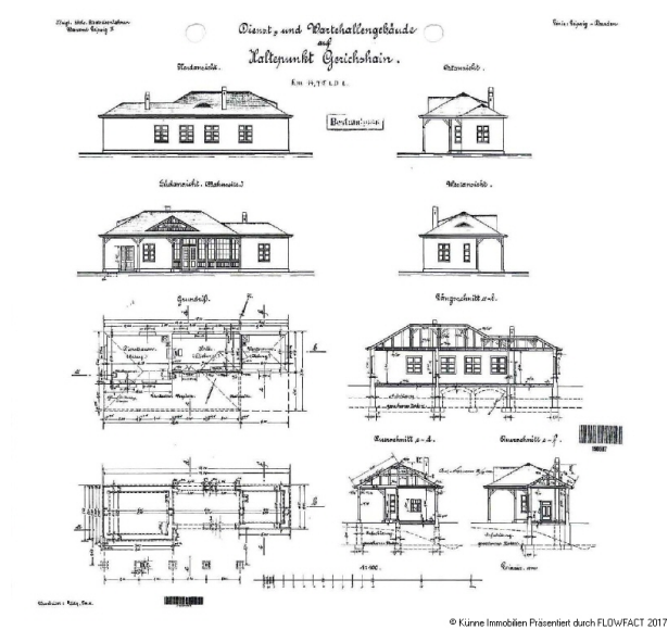
Grundrisse
