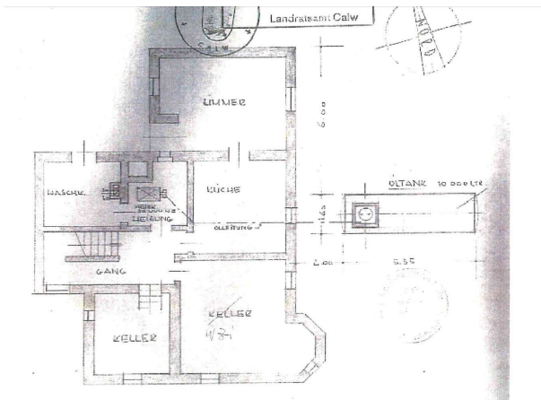
Grundriss Keller
