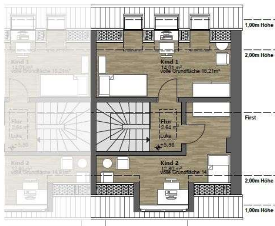
Dachgeschoss
