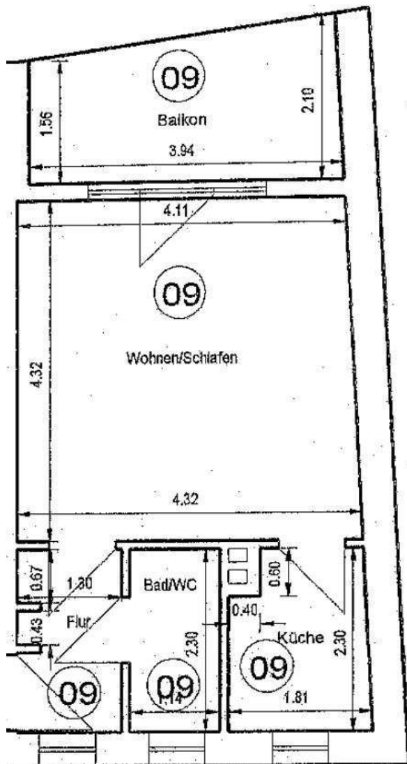
Grundriss WE9
