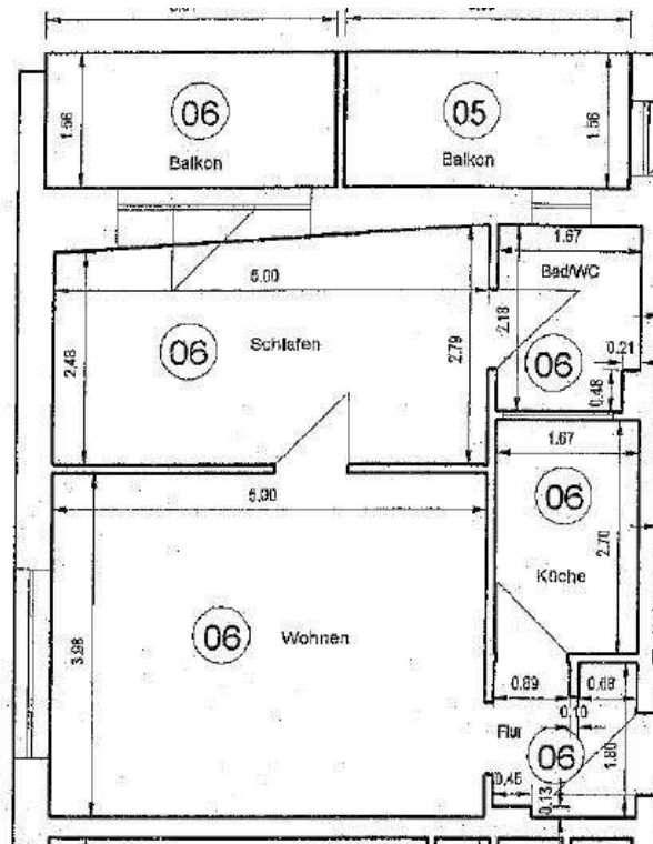
Grundriss WE06
