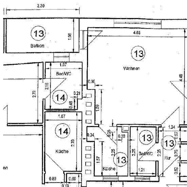
Grundriss WE13
