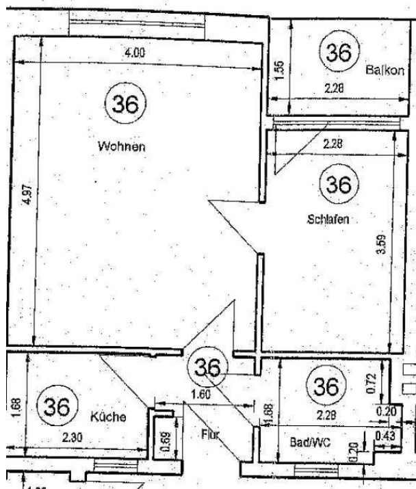
Grundriss WE36
