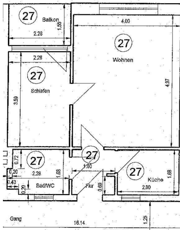
Grundriss WE27
