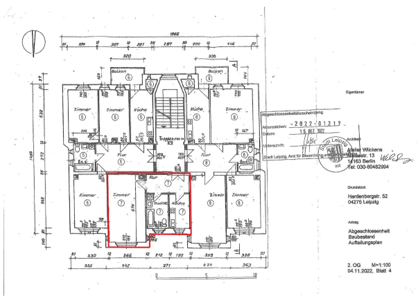
2.OG Mitte_Grundriss
