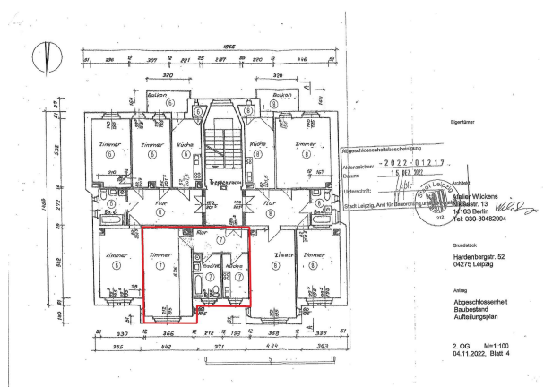
2.0G Mitte_Grundriss
