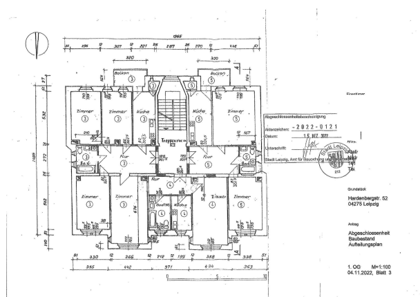
1.OG Grundriss
