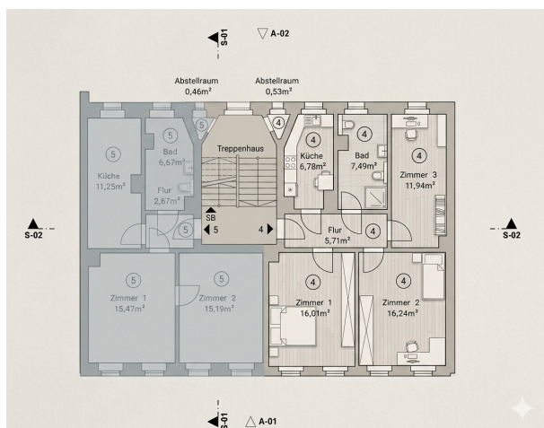
Grundriss
