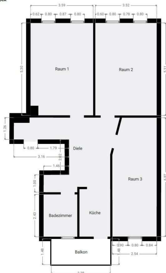
Grundriss 1.OG WE3
