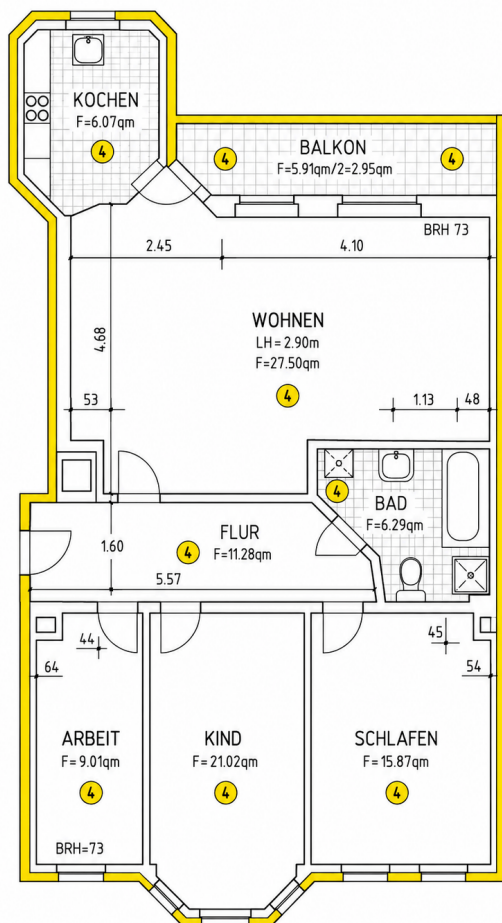
Grundriss WE4
