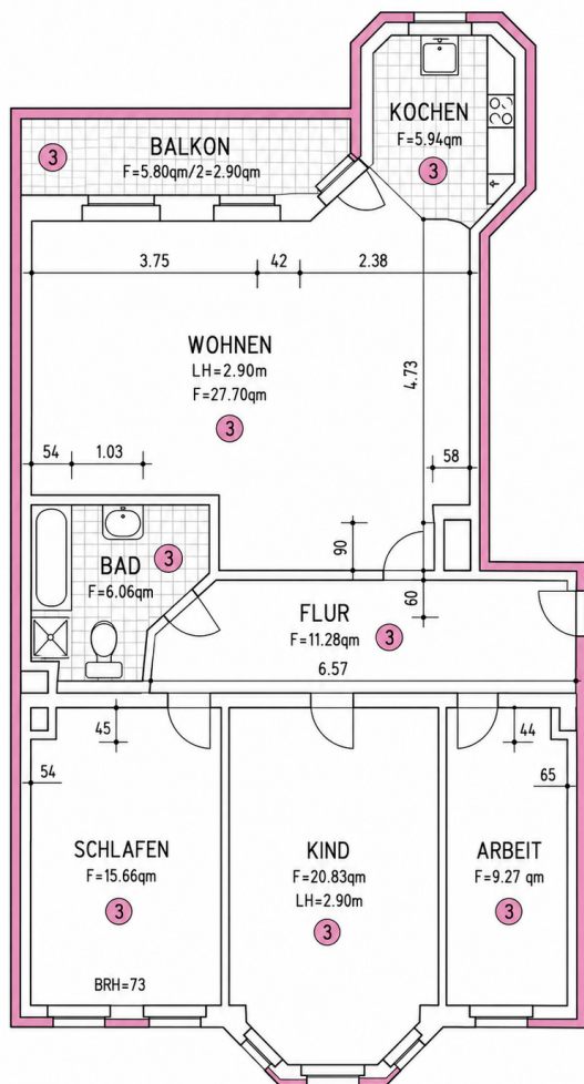
Grundriss WE3
