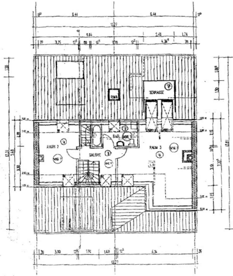
Grundriss 2. DG-Ebene
