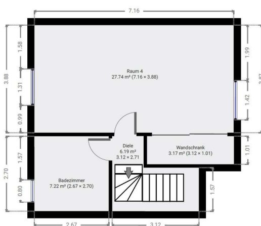
Grundriss 2
