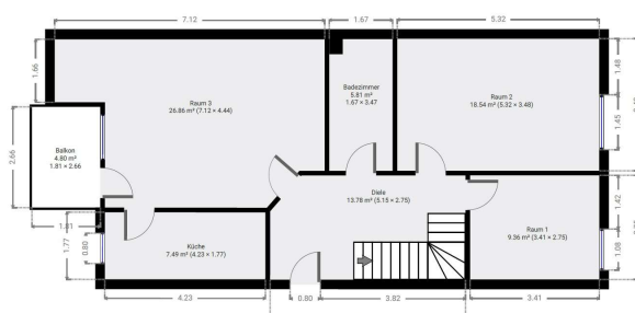
Grundriss 1
