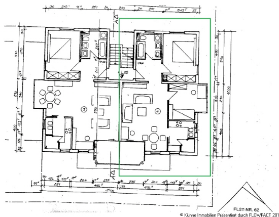
Grundriss WE 4
