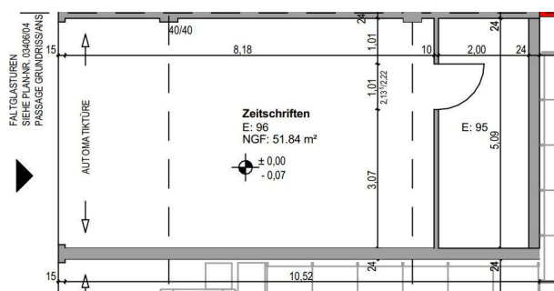
Grundriss
