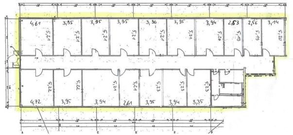
Grundriss 2.0GL
