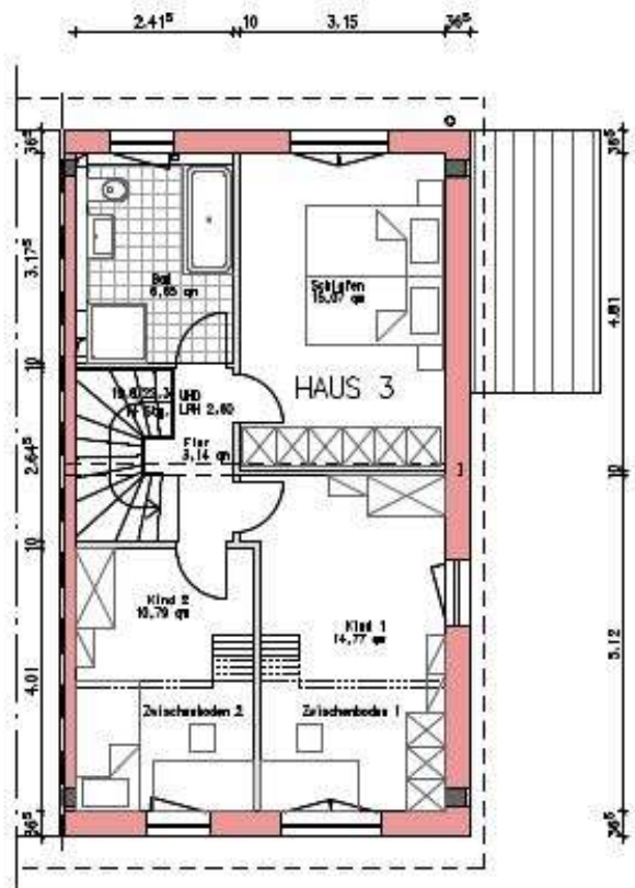
Grundriss OG
