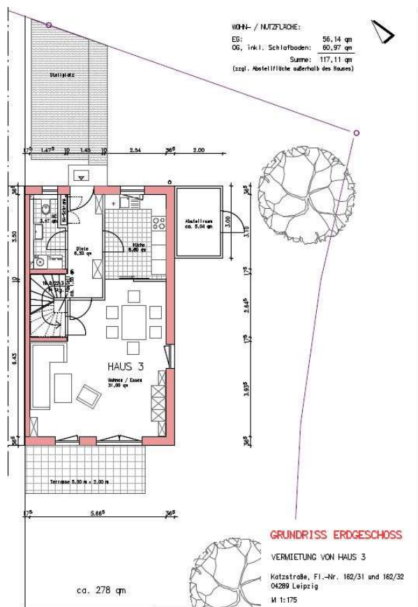
Grundriss EG
