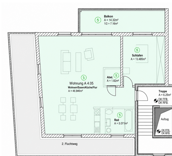
Grundriss
