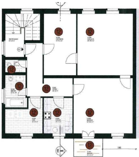
Grundriss 1.OG
