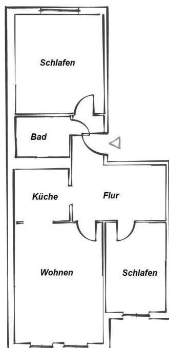
Grundriss
