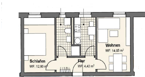
Grundriss 1C, 2.0GM
